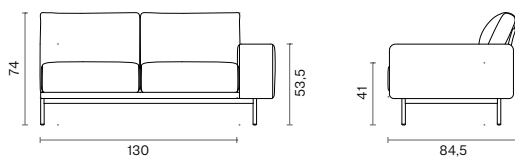
155 LEFT - 155L
