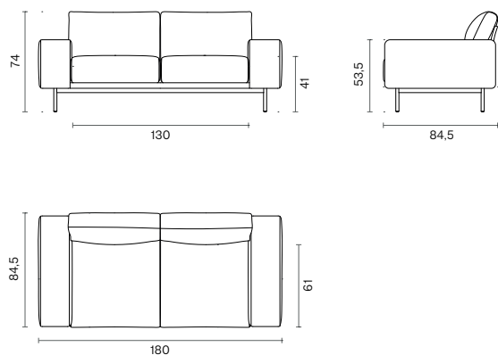
DOUBLE 180
