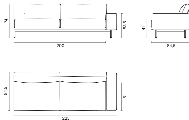
225 LEFT - 225L
